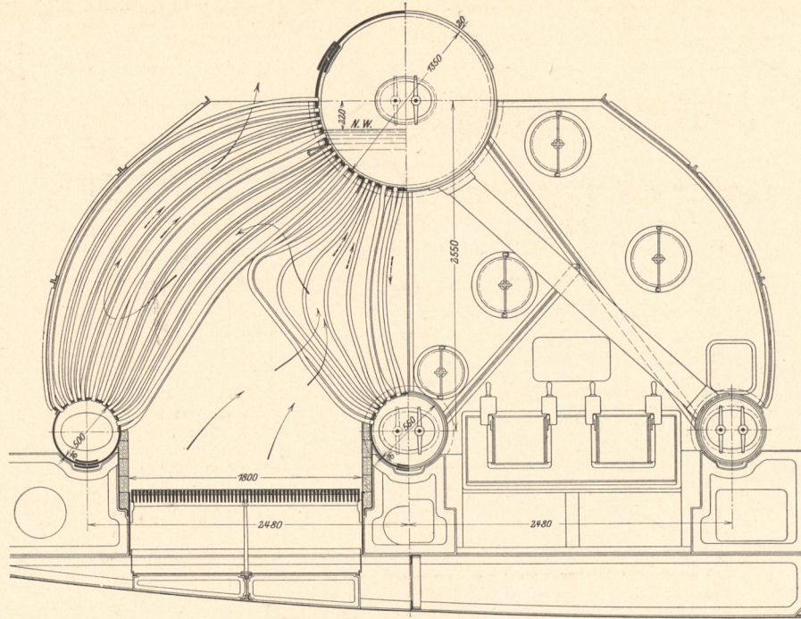
Fig. 126. Doppellendiger Wasserrohrkessel (Patent R. Schulz).
