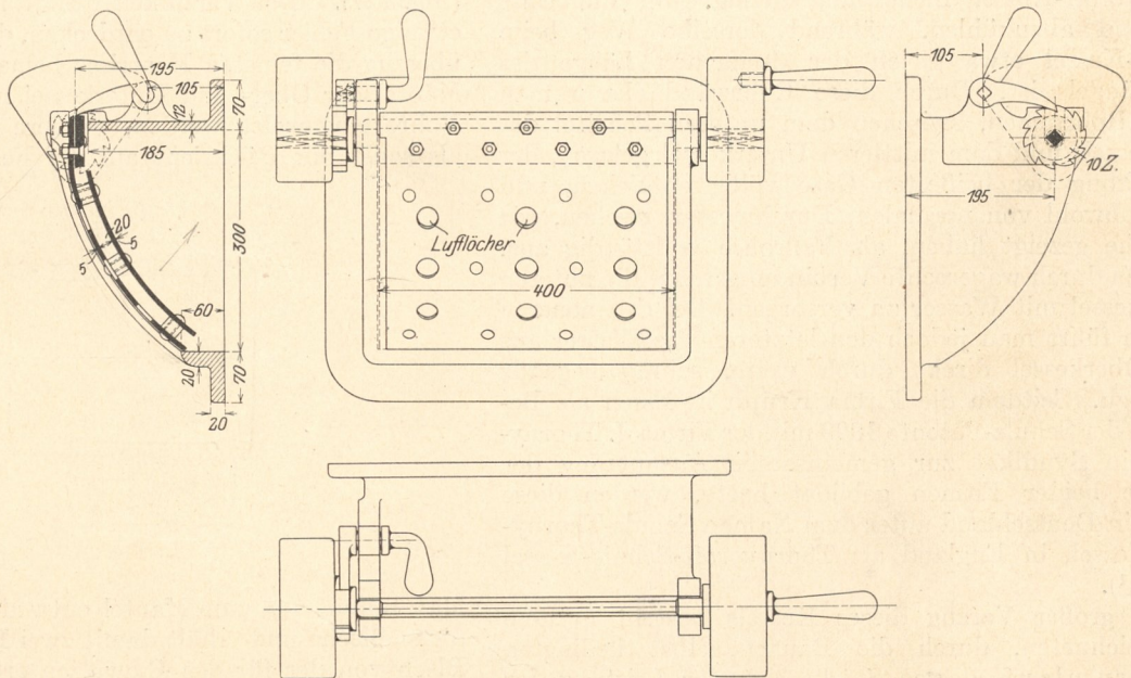
Fig. 125. Kipptür zum Schiffskessel, Fig. 123.
