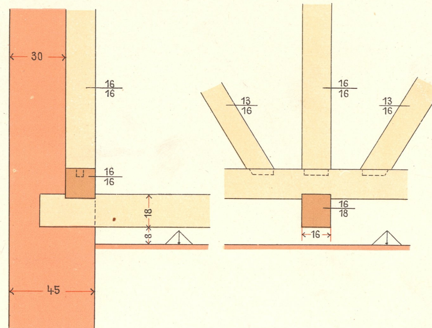
Einzelheiten bei der Riegelwand (Hochwand)
