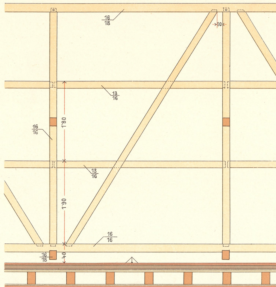
Längenschnitt ohne Sparren.
