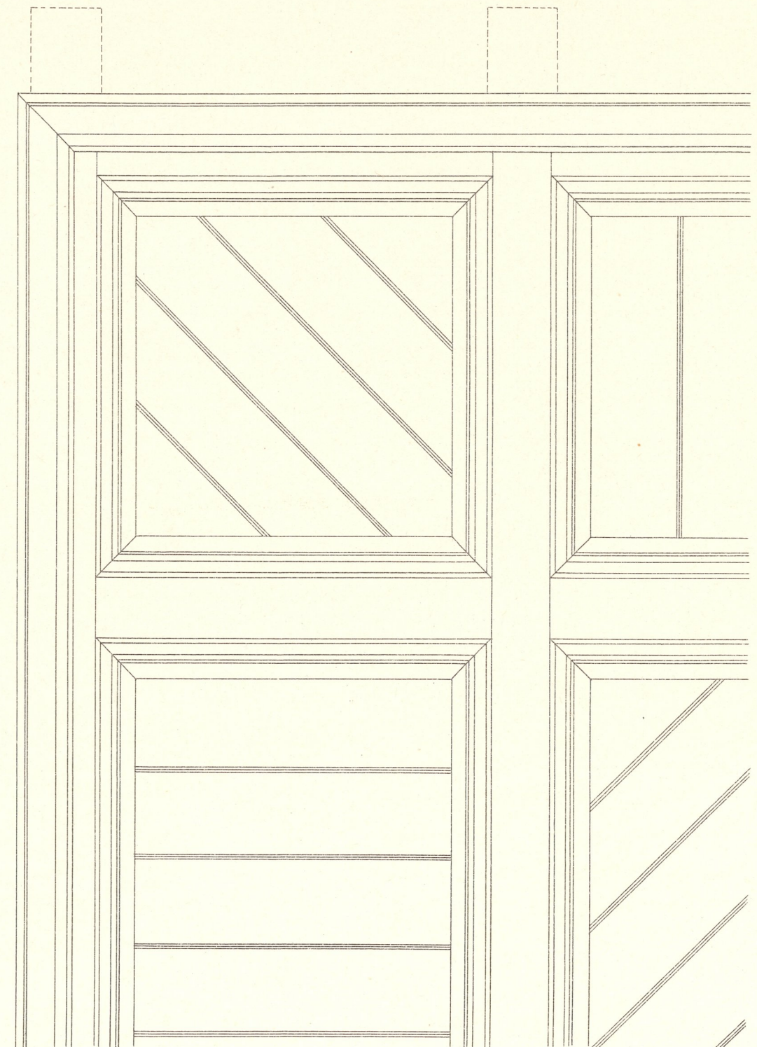
Druntersicht mit diagonal verschaltem Eckfeld.
