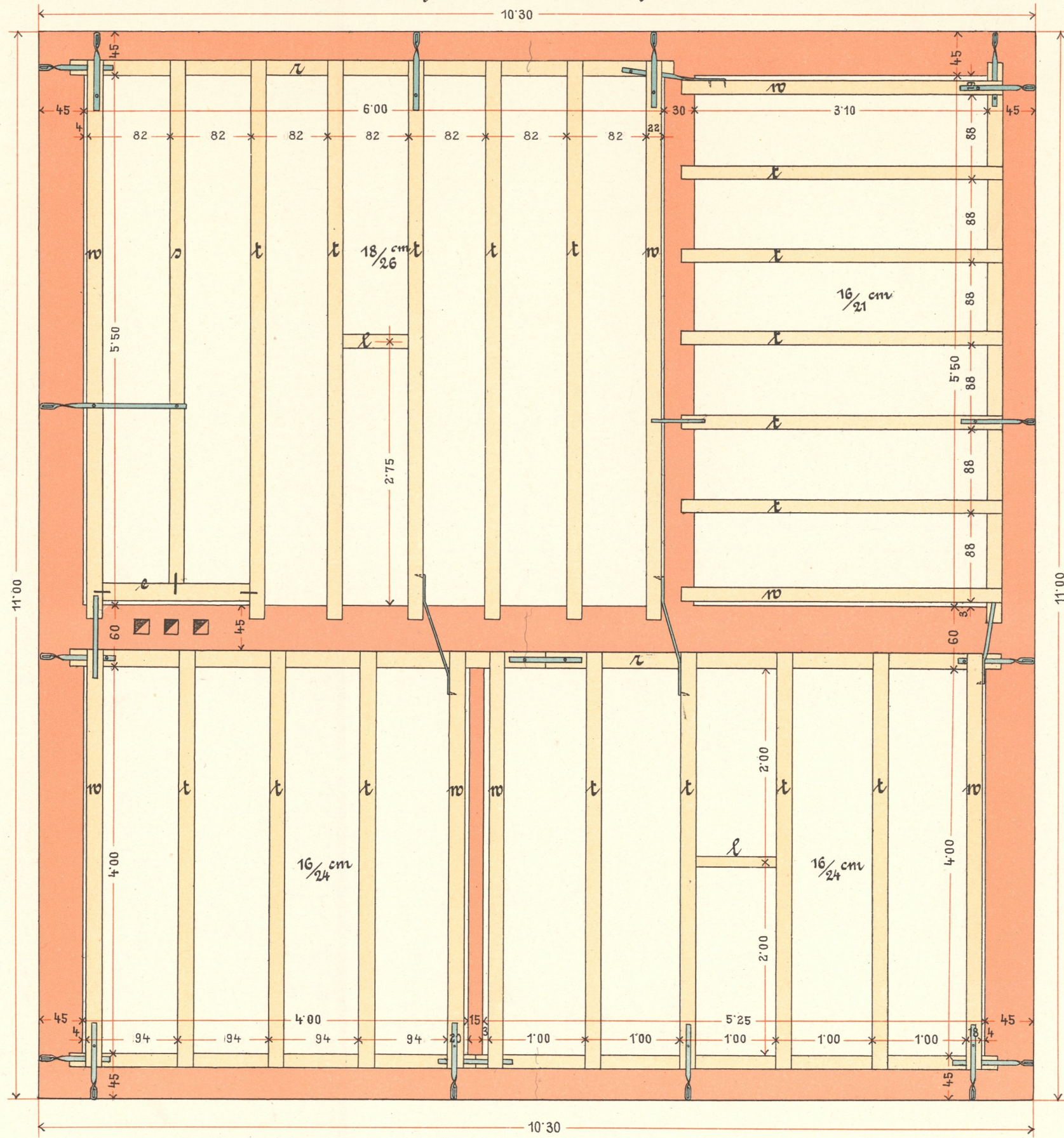
Tramlage in einem Wohngebäude.
