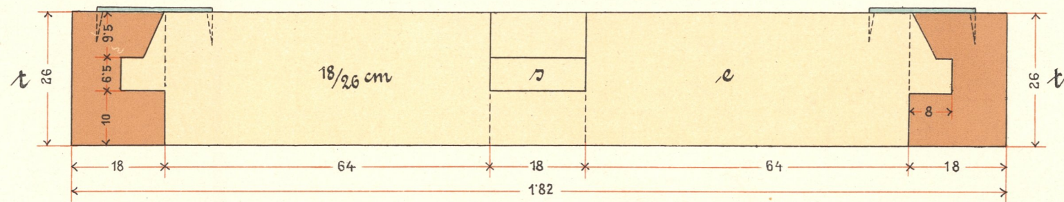
Tramauswechslung beim Rauchfang.
