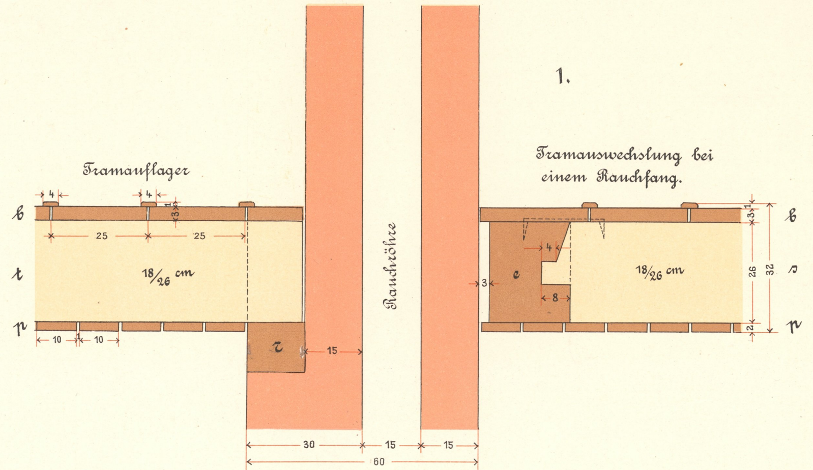
Einzelheiten des Trambodens.
