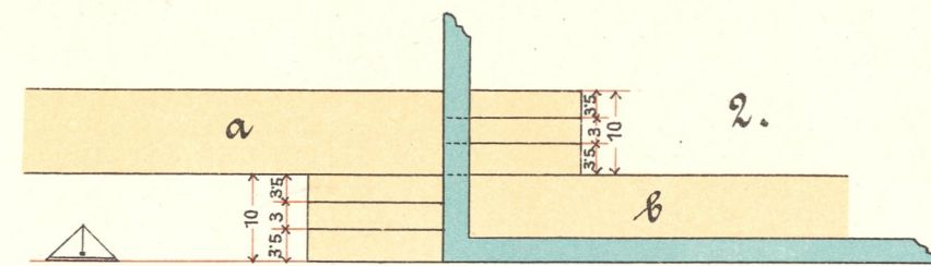
Einzelheiten bei der Sparrenkupplung
