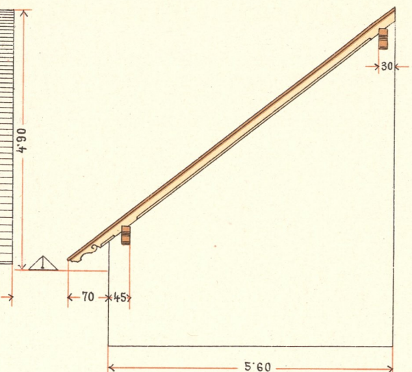
Giebelansicht
