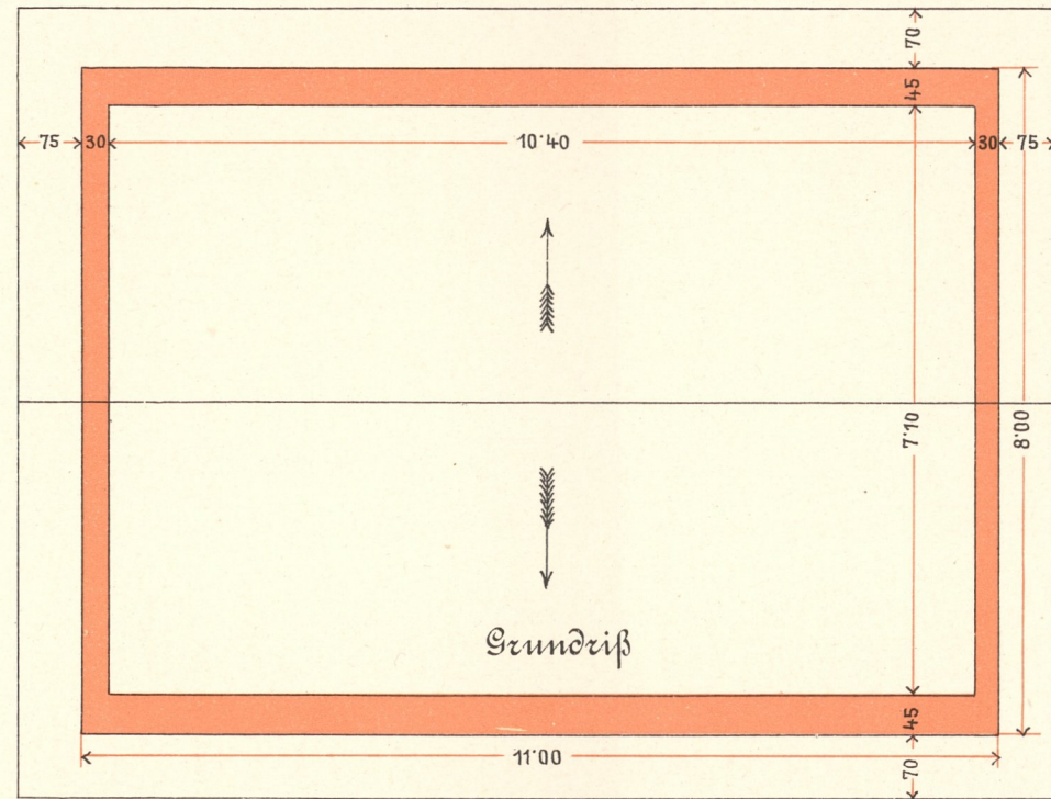
Satteldach mit Giebel.
