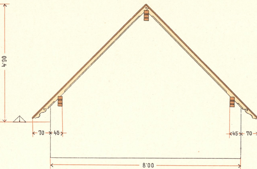
Giebelansicht
