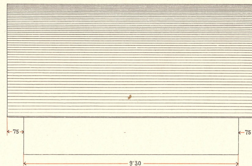
Seitenansicht
