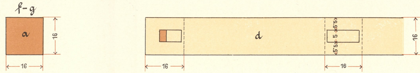
Verzapfung der Säule mit Schwelle und Pfette.
