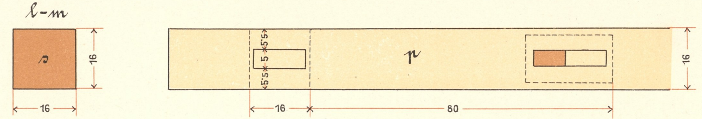
Verzapfung des Kopfbandes mit Säule und Pfette.
