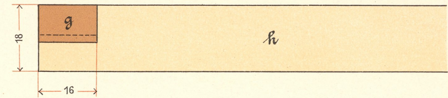
Hakenförmige Überblattung am Eck.
