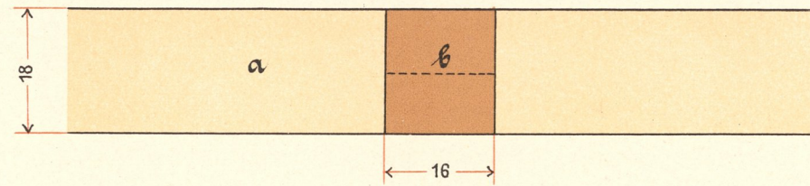
Gerade Überblattung.
