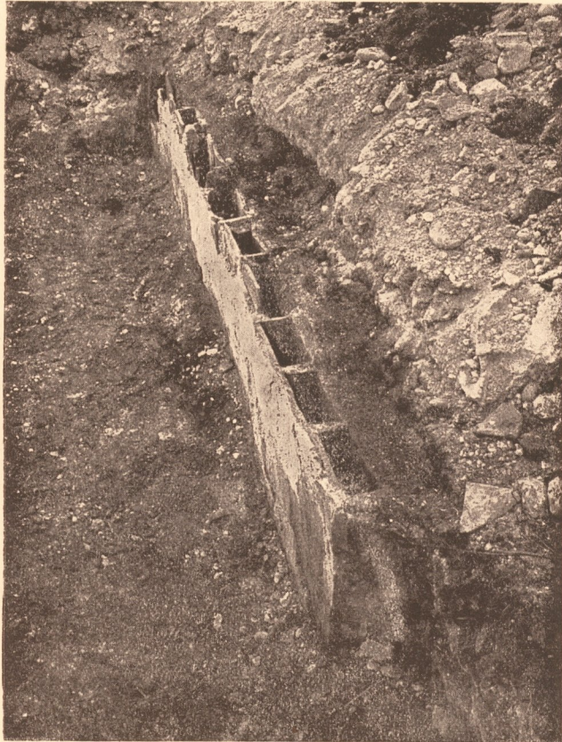
Abb. 51. Viereckige Hohlziegel in der aufgehenden Wand, die in Verbindung mit der Heizanlage standen und die Wand erwärmten.
