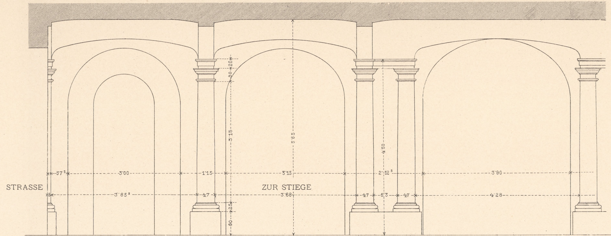
LÄNGENSCHNITT NACH A. B.
