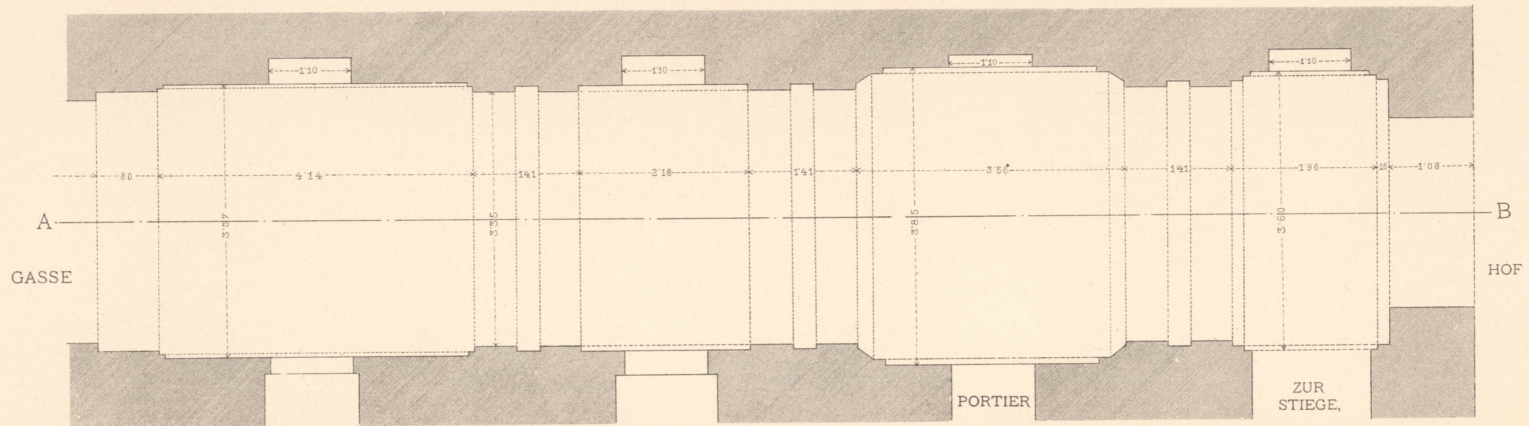
GRUNDRISS
