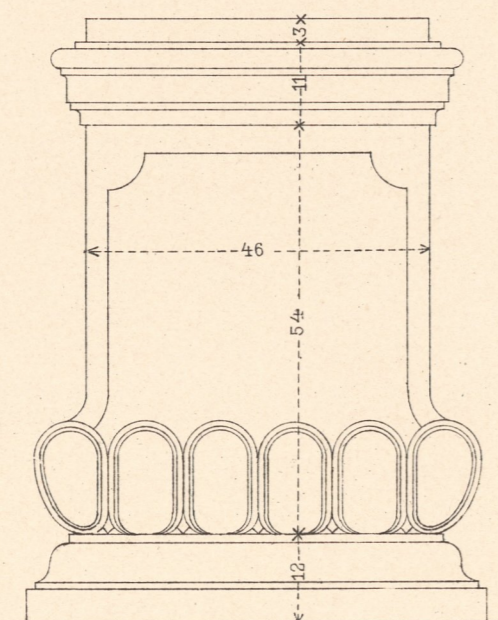
DETAIL DES POSTAMENTES IM STIEGENHAUS.
