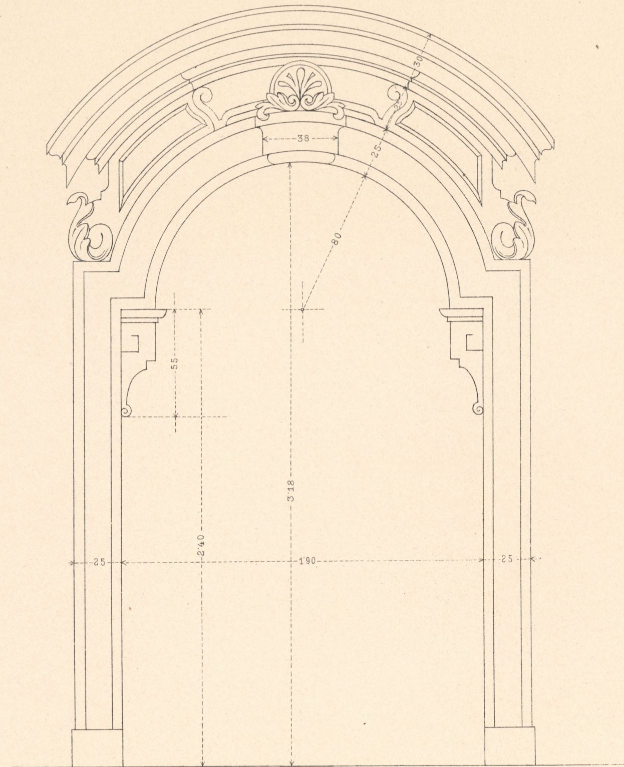
THÜR IM VESTIBUL.
