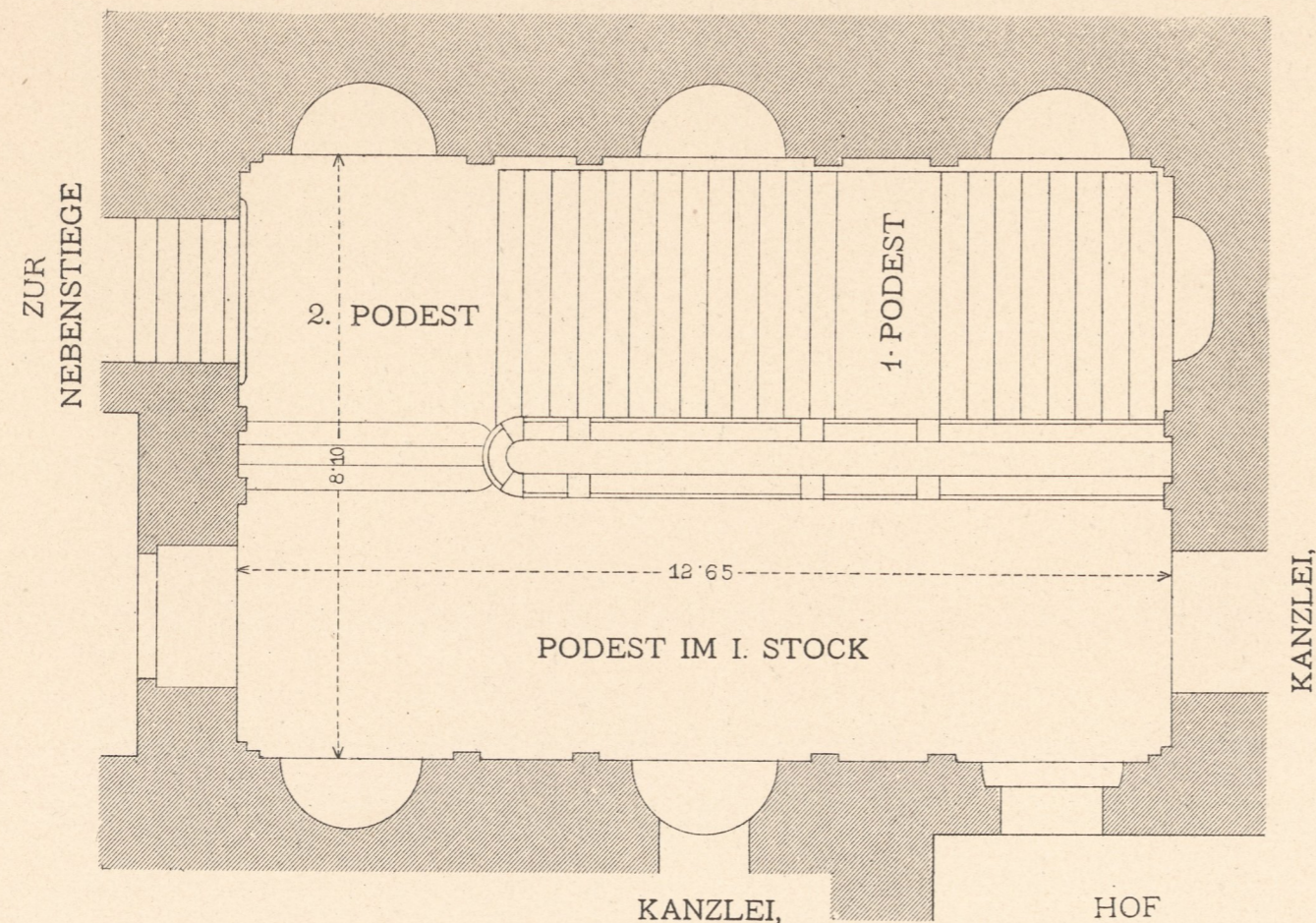
GRUNDRISS DES STIEGENHAUSES IM 1. STOCK.
