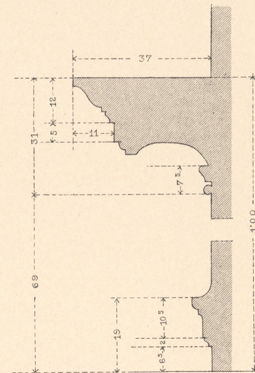
GESIMS ÜBER DEN PILASTERN
