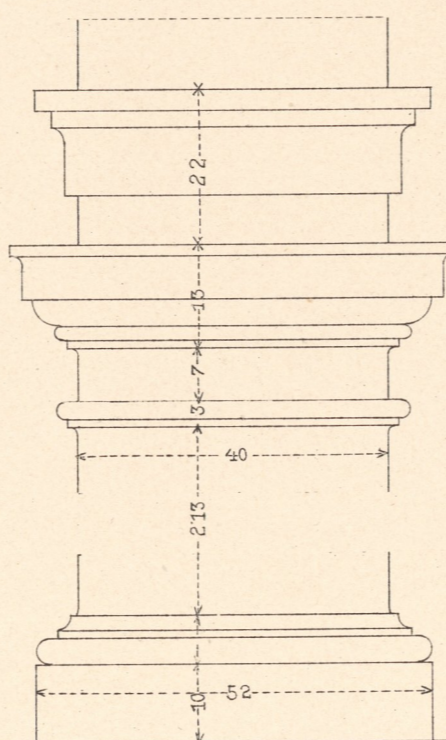
DETAIL DER PILASTER IM VESTIBUL.
