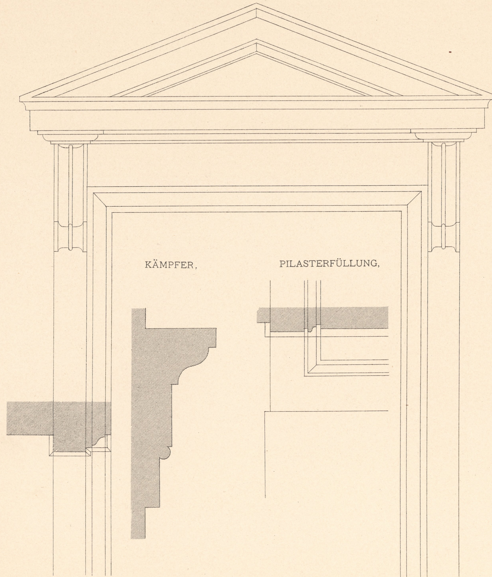
DETAIL DER THÜRE IM VESTIBUL
