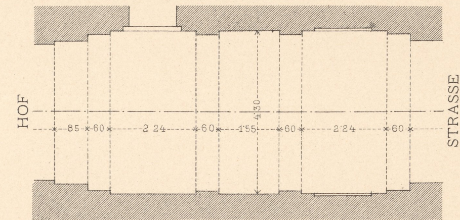
GRUNDRISS DES VESTIBULS IM HAUSE
