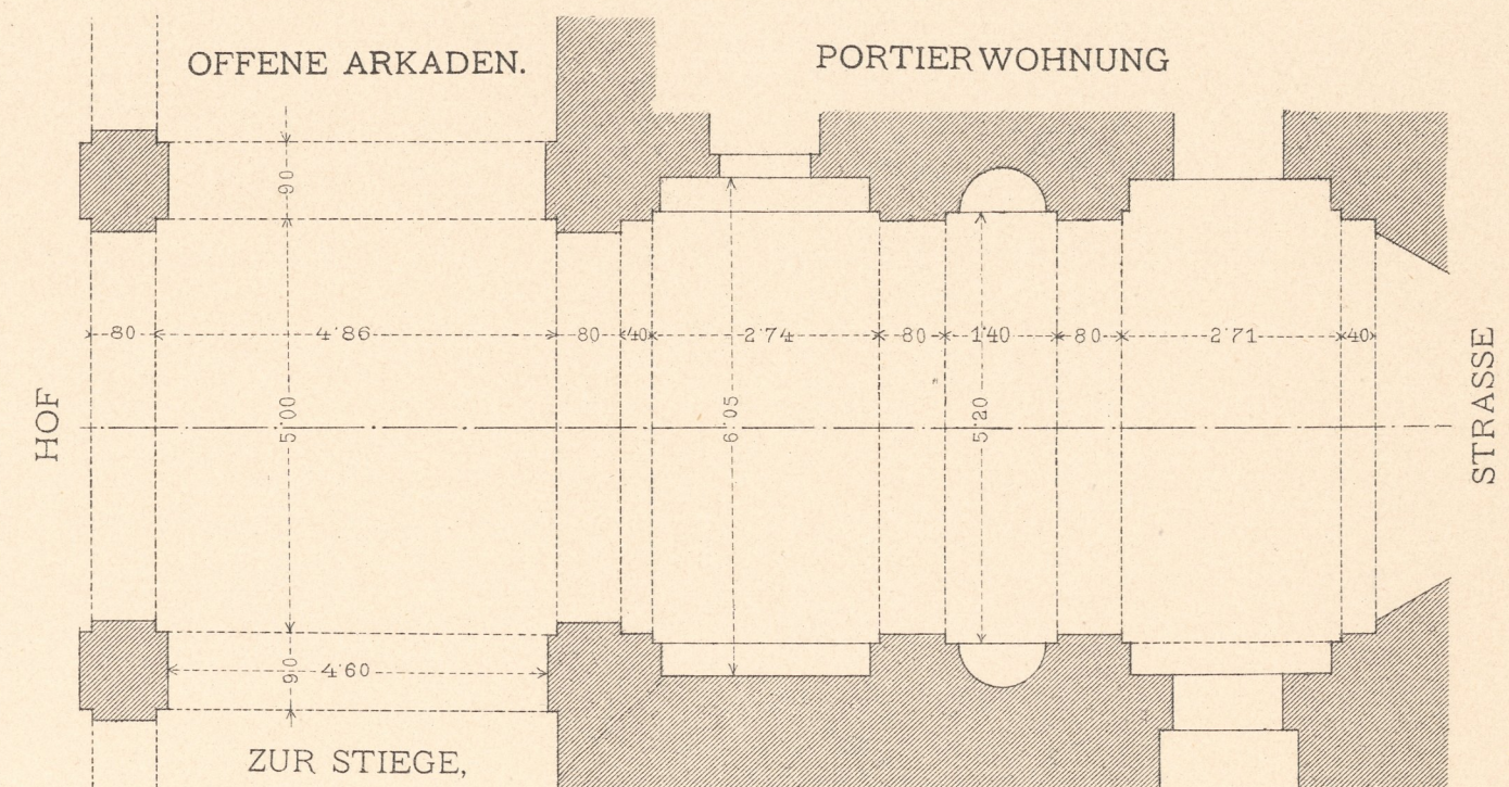
GRUNDRISS DES VESTIBULS IM HAUSE
