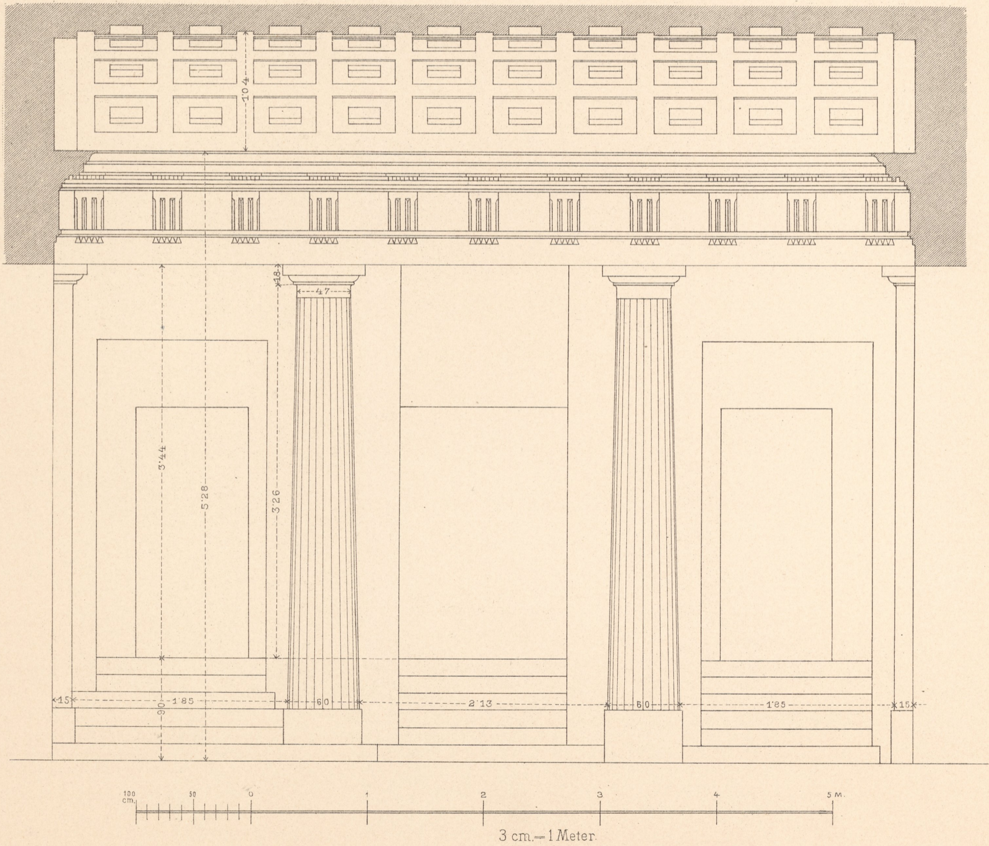
QUERSCHNITT NACH C. D.
