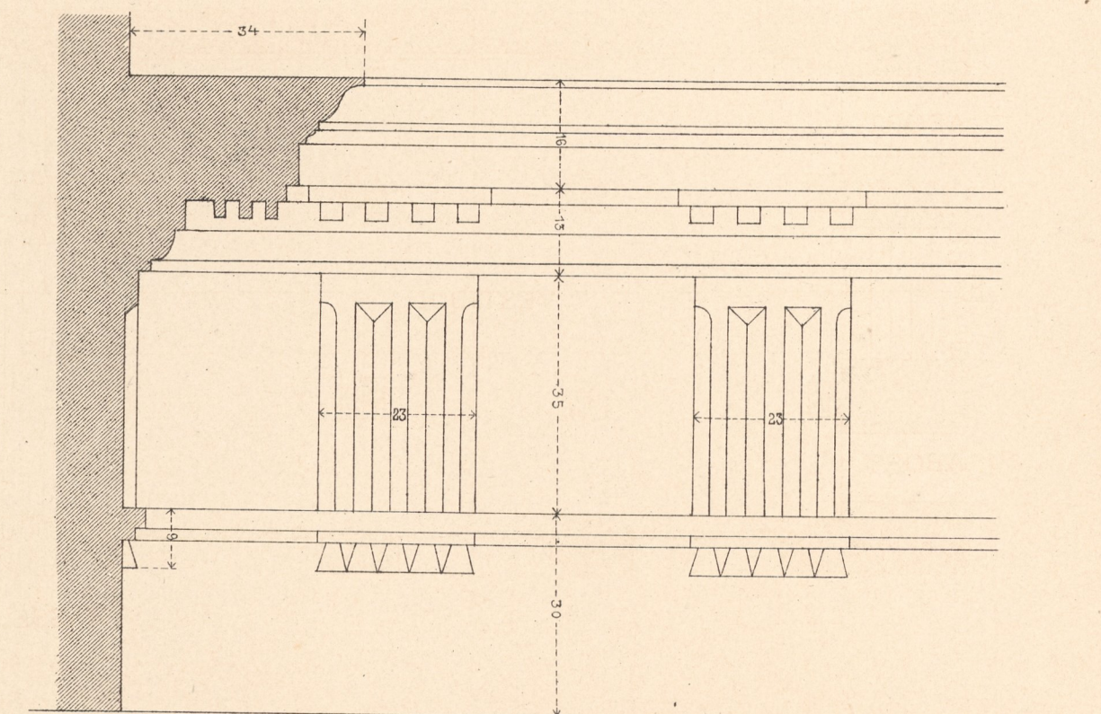
GESIMS IN DER EINFÄHRT.
