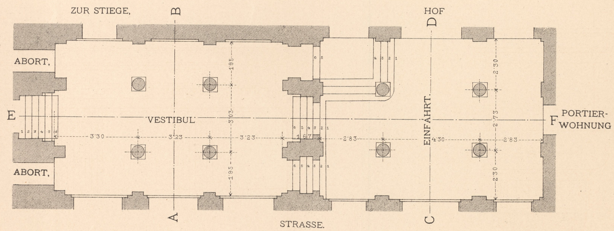
GRUNDRISS
