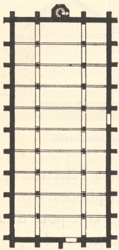
Fig. 1358. — Grange de l'abbaye de Maubuisson.
