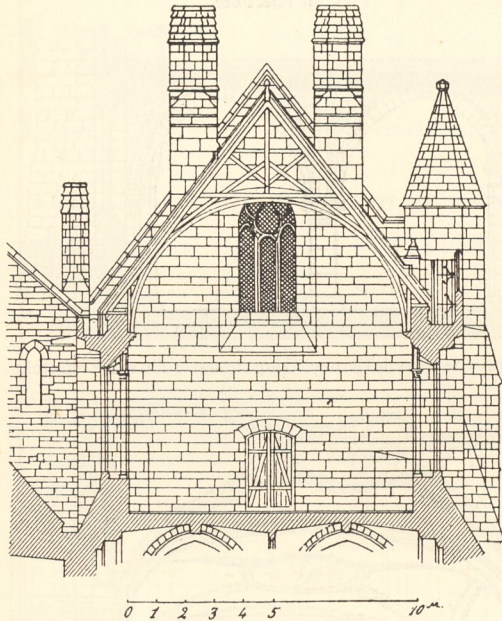
Fig. 1357. — Dortoir du Mont-Saint-Michel. Coupe transversale.
