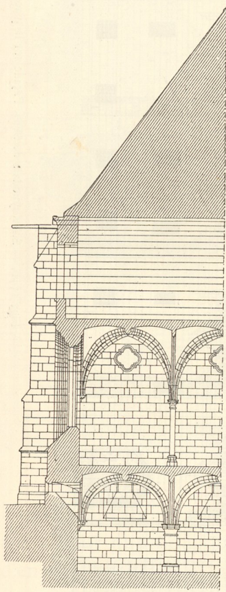
Fig. 1353. — Collège des Bernardins, à Paris. Coupe transversale du réfectoire.
