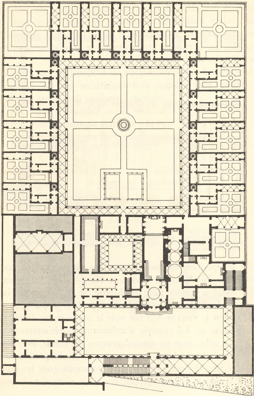
Fig. 1346. — Chartreuse de Florence. Plan.
