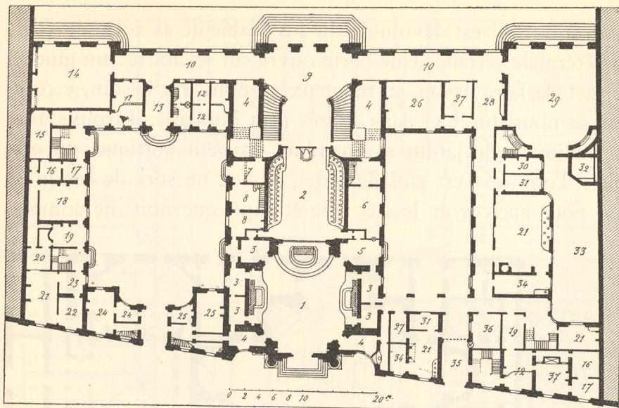
Fig. 1343. — Ancienne abbaye de Pantemont, à Paris. Plan du rez-de-chaussée.
