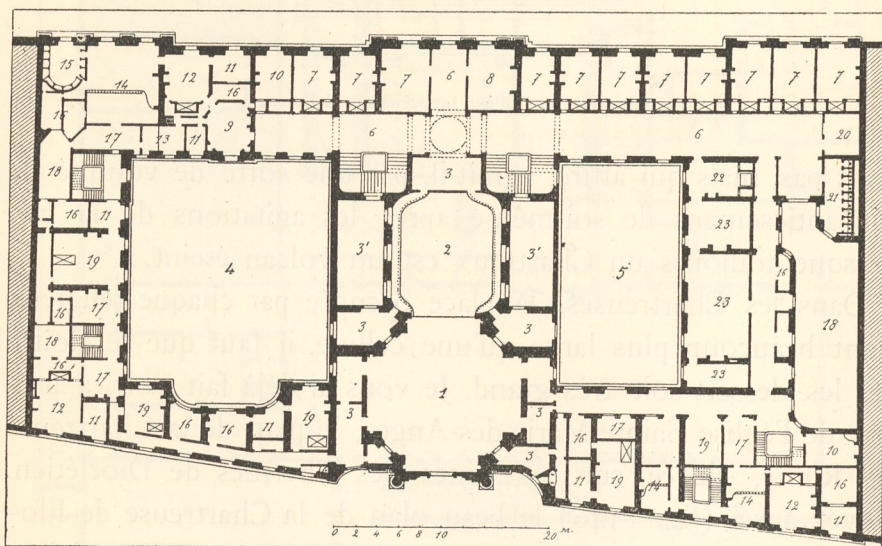
Fig. 1344. — Ancienne abbaye de Pantemont, à Paris. Plan du 1 er étage.
