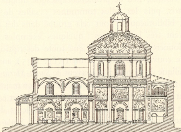
Fig. 1337. — Couvent de Santa Maria della Pace, à Rome. Coupe longitudinale.
