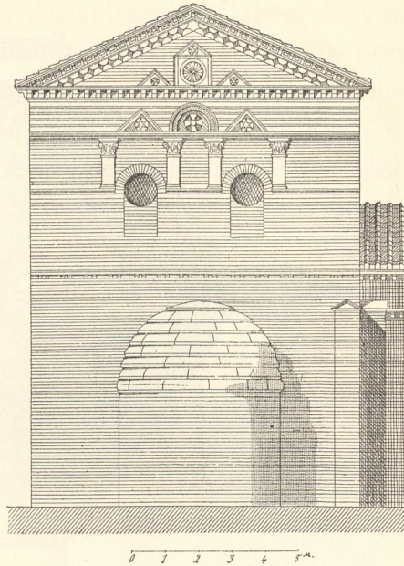
Fig. 1233. — Baptistère Saint-Jean, à Poitiers. Façade.
