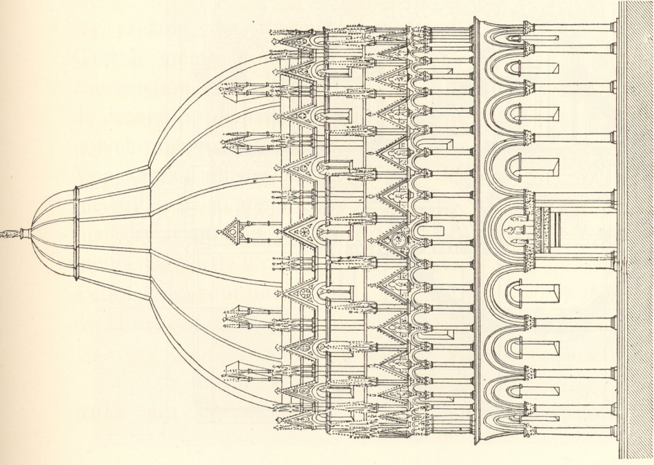
Fig. 1228. — Baptistère de Pise. Façade.
