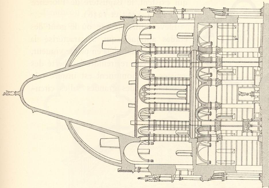
Fig. 1229. — Baptistère de Pise. Coupe.
