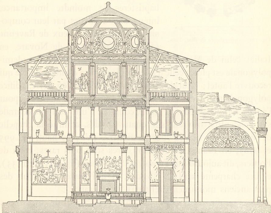
Fig. 1226. — Baptistère de Constantin. Coupe.
