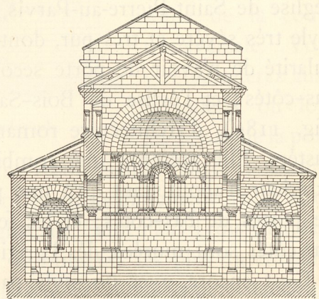
Fig. 1186. — Église de Loupiac. Coupe transversale.
