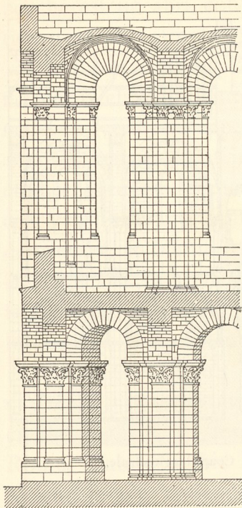
Fig. 1172. — Porche engagé de l'église de Saint-Benoit-sur-Loire.
