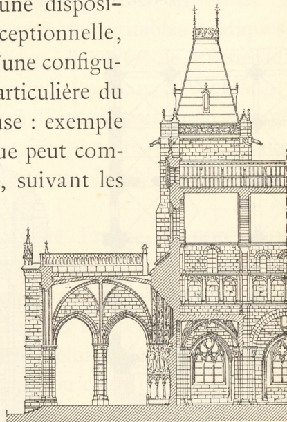
Fig. 1174. — Église Notre-Dame, à Beaune. Coupe longitudinale.
