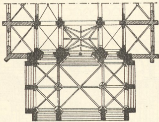
Fig. 1173. — Église de Notre-Dame de Beaune. Plan.
