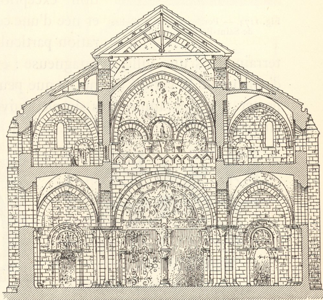
Fig. 1170. — Église de la Magdeleine, à Vézelay. Coupe transversale
