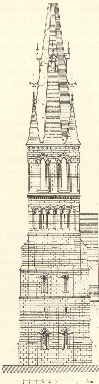
Fig. 1167. — Flèche de l'église de Montier-en-Der.
