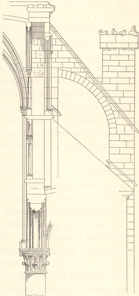
Fig. 1075. — Nef de Notre-Dame de Dijon. Coupe.
