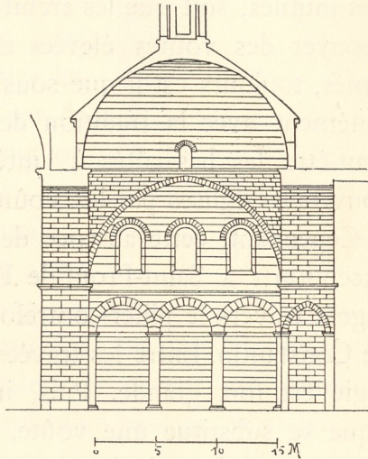
Fig. 1030. — Église de Cahors. Coupe transversale.
