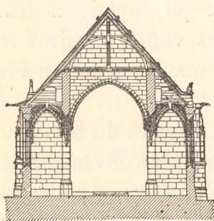
Fig. 965. — Église d'Appeville. Coupe transversale.
