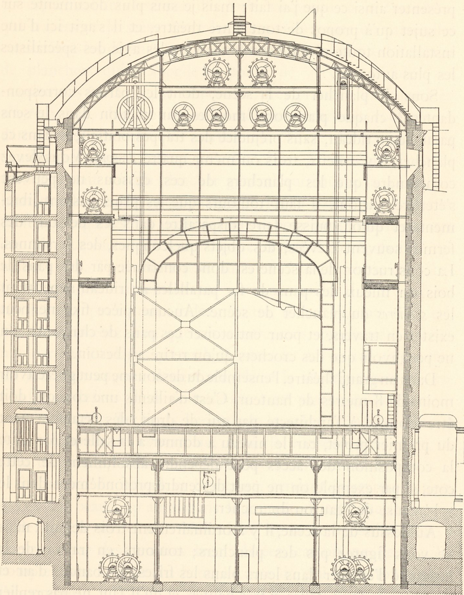
Fig. 905. — Coupe transversale de la scène du Théâtre-Français.
