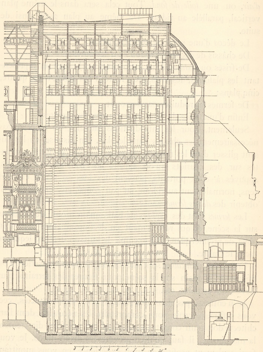
Fig. 904. — Coupe longitudinale de la scène.
