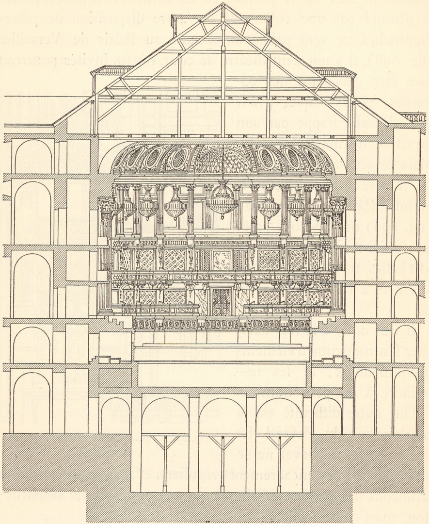
Fig. 898. — Coupe transversale de la salle de l'Opéra de Versailles.
