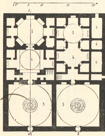
Fig. 876. — Bains turcs à Constantinople. Plan et coupe.
