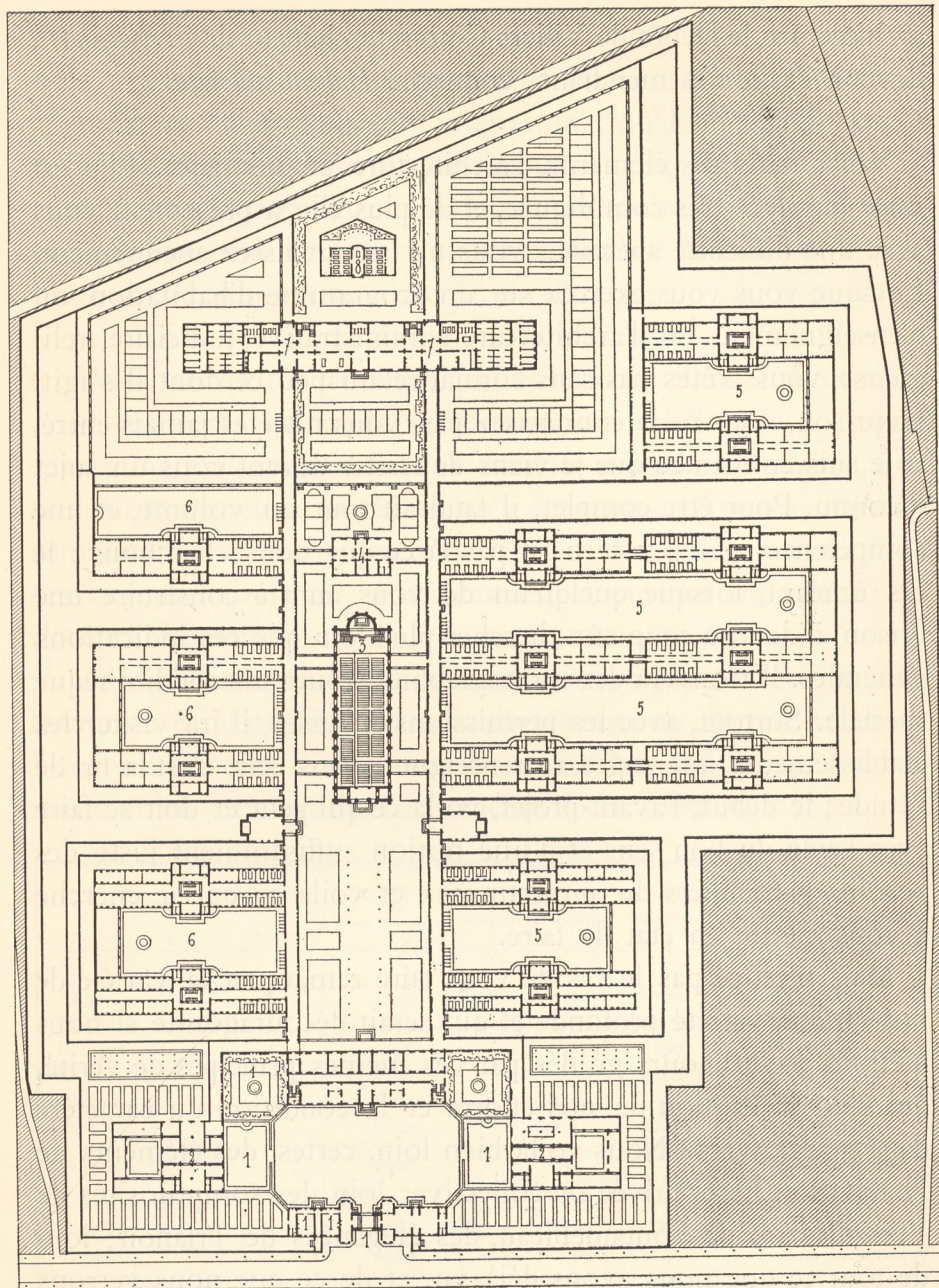
Fig. 814. — Maison de répression de Nanterre. Plan général.
