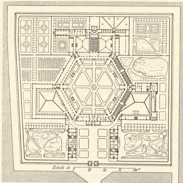
Fig. 810. — Maison centrale de Rennes. Plan du rez-de-chaussée.
