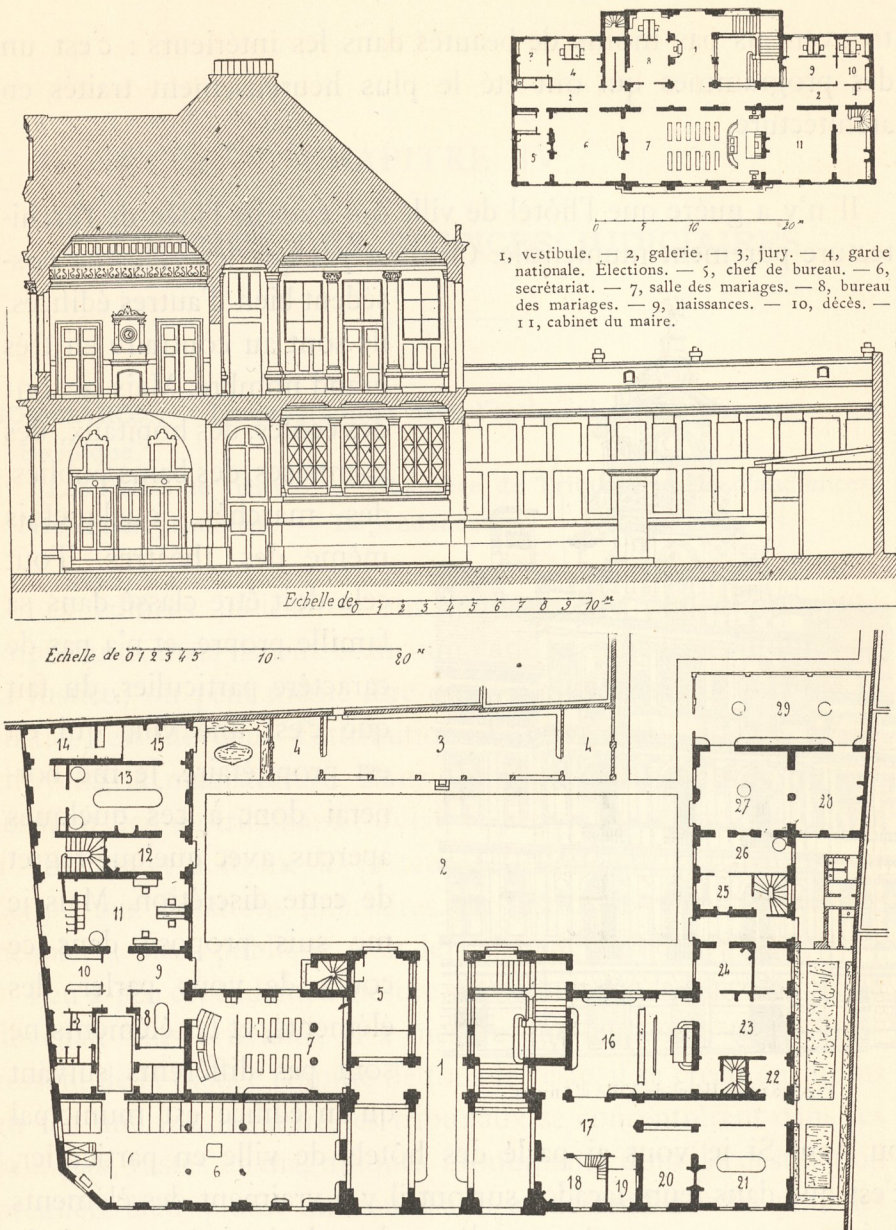
Fig. 781. — Mairie de Saint-Sulpice, à Paris (avant ses agrandissements). Plan du rez-de-chaussée et coupe.
