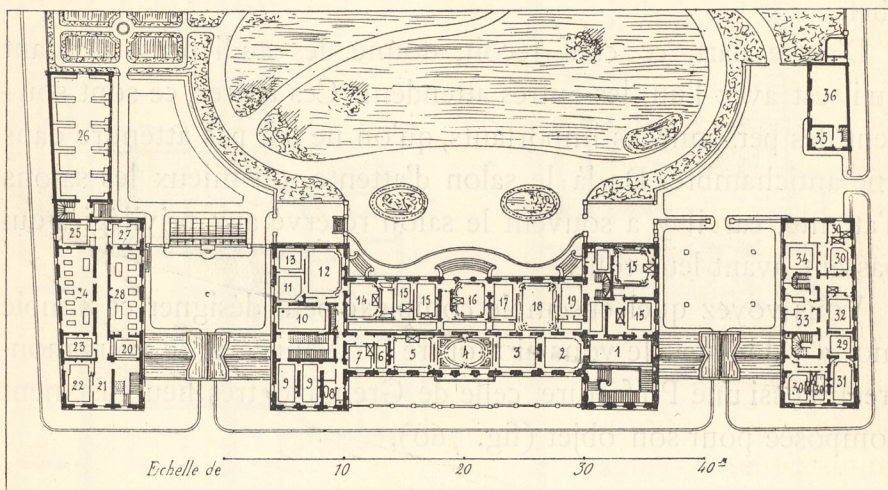
Fig. 760. — Préfecture de Grenoble. Plan du 1 er étage.
