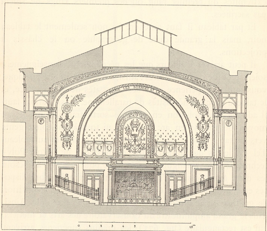
Fig. 671. — Coupe transversale de l'amphithéâtre de l'École Polytechnique.
