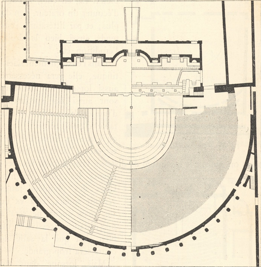
Fig. 668. — Plan du grand théâtre de Pompéi.
