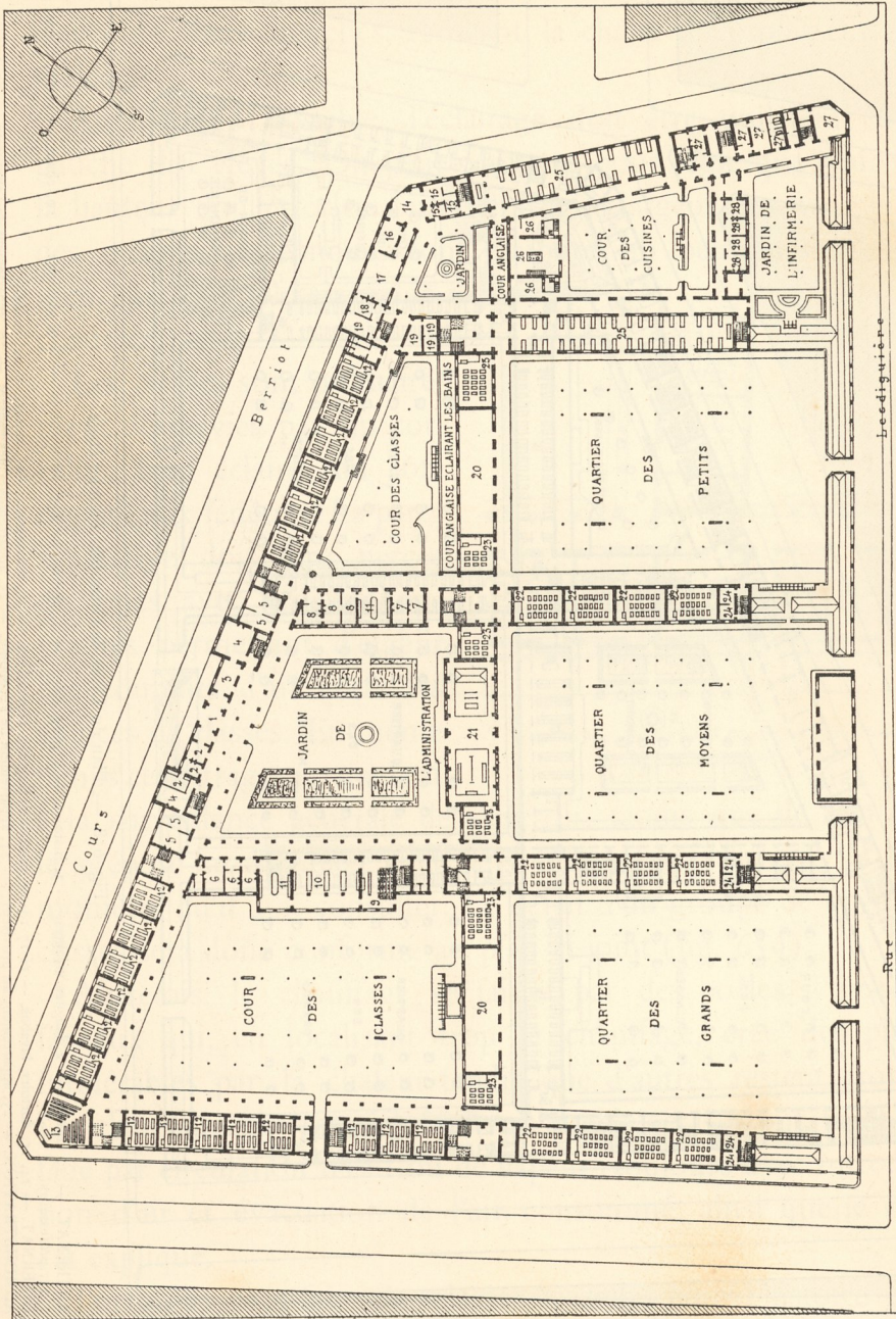
Fig. 657. — Plan du Lycée de Grenoble. Rez-de-chaussée. EXTERNAT. — 1-2, entrée, conciergerie. — 3-4, parlours. — 5, professeurs. — 6-7-8, direction. — 9-10, histoire naturelle. — 11, bibliothèque. — 12, classes. — 13, chant. — 14-15, entrée et conciergerie des petits. — 16-17, parlours. — 18-19, économat. INTERNAT. — 20, préau. — 21, gymnase. — 22-23, études. — 24, musique. — 25, réfectoires — 26, cuisine. — 27-28, service médical.
