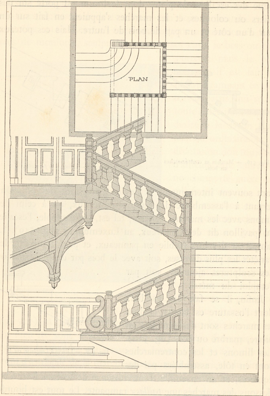
Fig. 519. — Escalier du Pavillon des Chartreux au Luxembourg. (D'après un relevé de M. Scellier de Gisors.)
