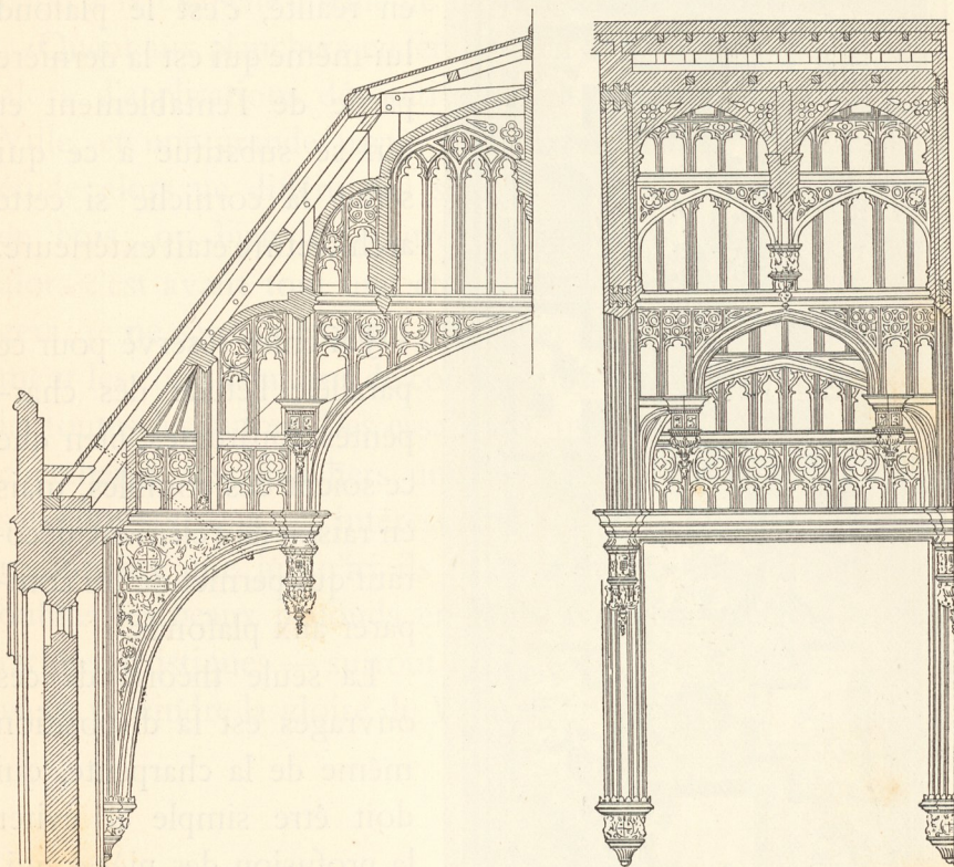
Fig. 426. — Charpente apparente de Hampton-Court (Angleterre).
