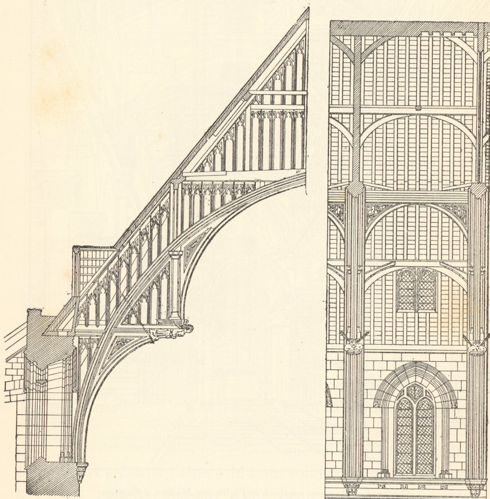
Fig. 425. — Charpente apparente de Westminster-Hall (Angleterre).
