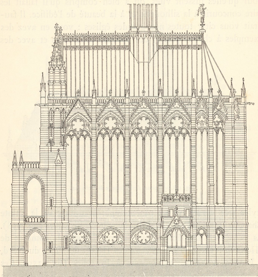
Fig. 357. — Toitures de la Sainte Chapelle.
