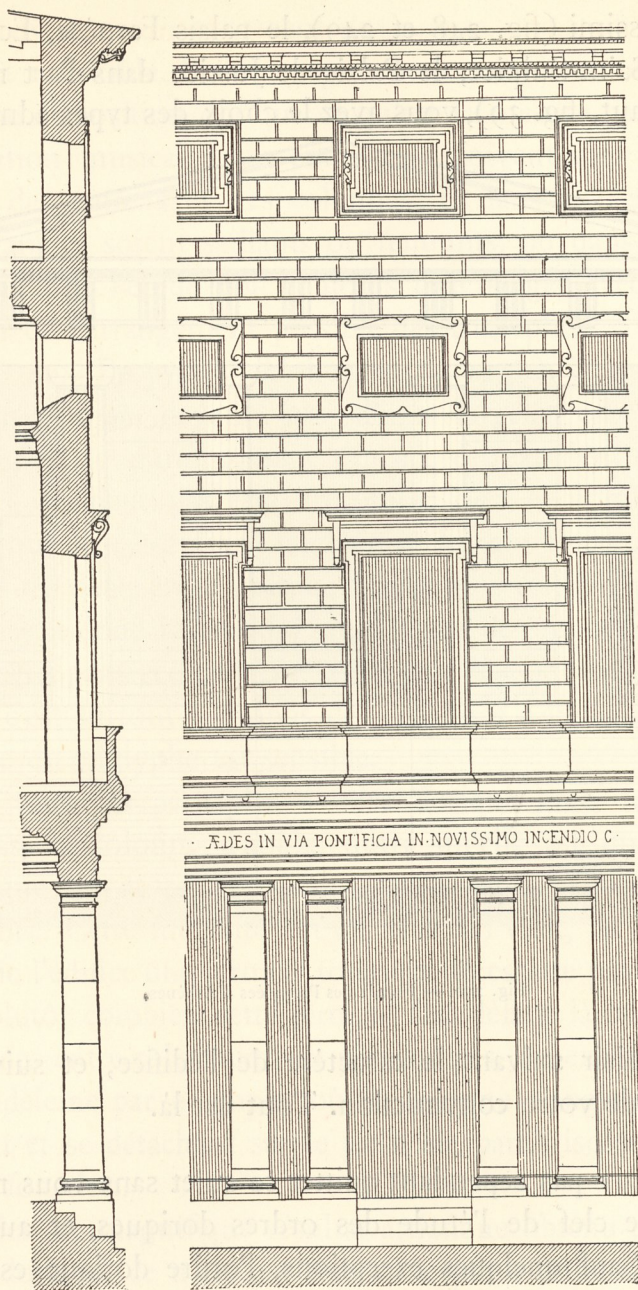
Fig. 249. — Palais Massimi. Travée. Élévation.
