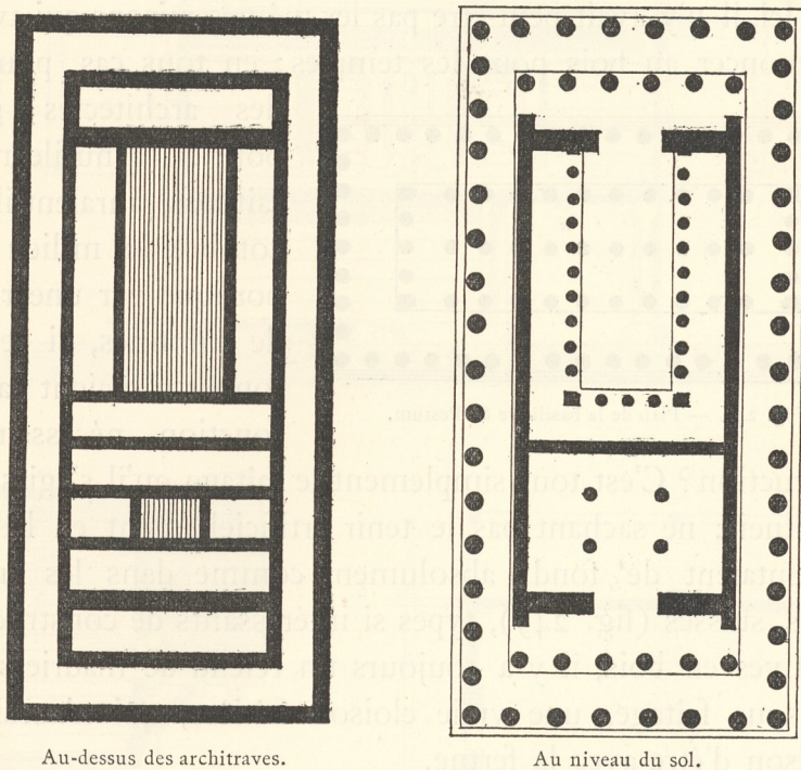
Fig. 243. — Plans du Parthénon.
