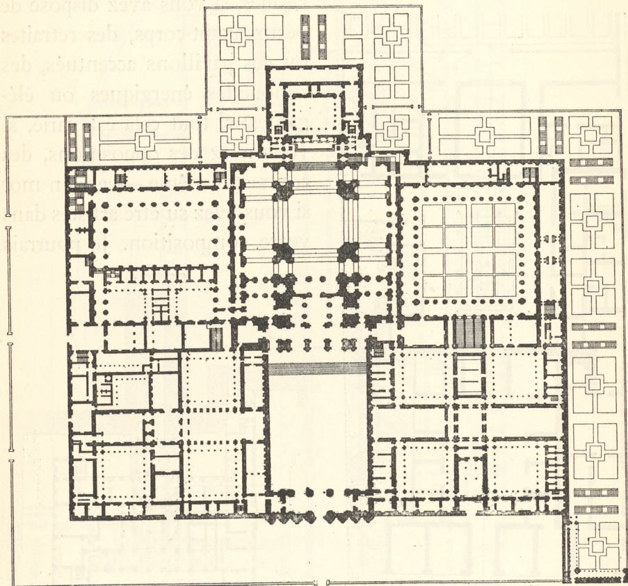
Fig. 35. — Plan de l'Escorial. Rez-de-chaussée.
