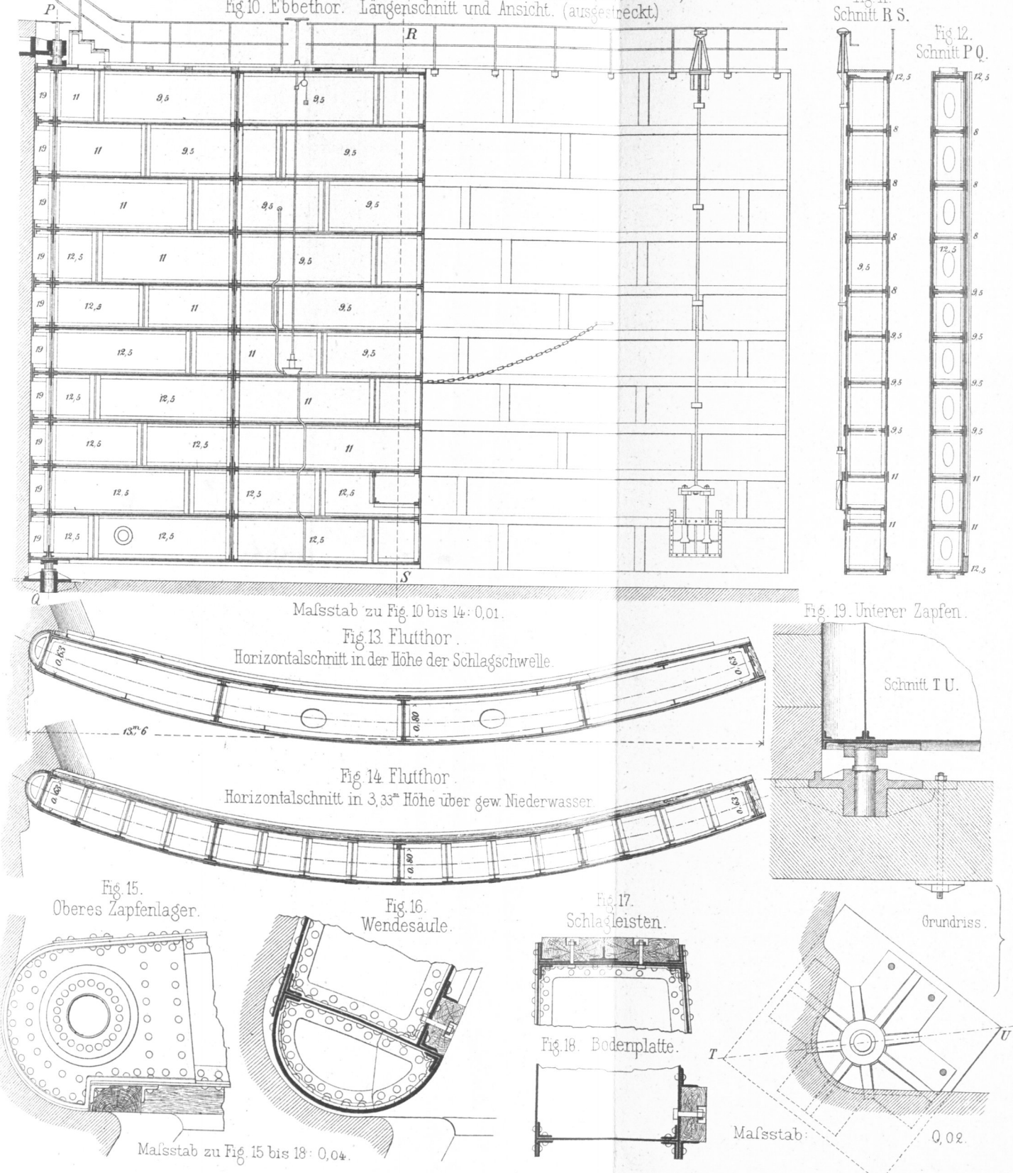
Fig 10 bis 19. Schleuse des Hafenbassins zu Geestemünde. (23,94 m weit)
