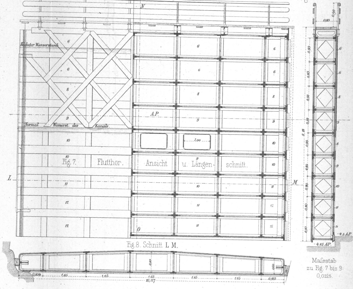
Fig 7 bis 9. Schleuse des Amsterdamer Nordsee-Kanals. (18,0 weit).
