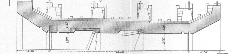
Maßstab zu Fig. 11 bis 14: 0,005.
