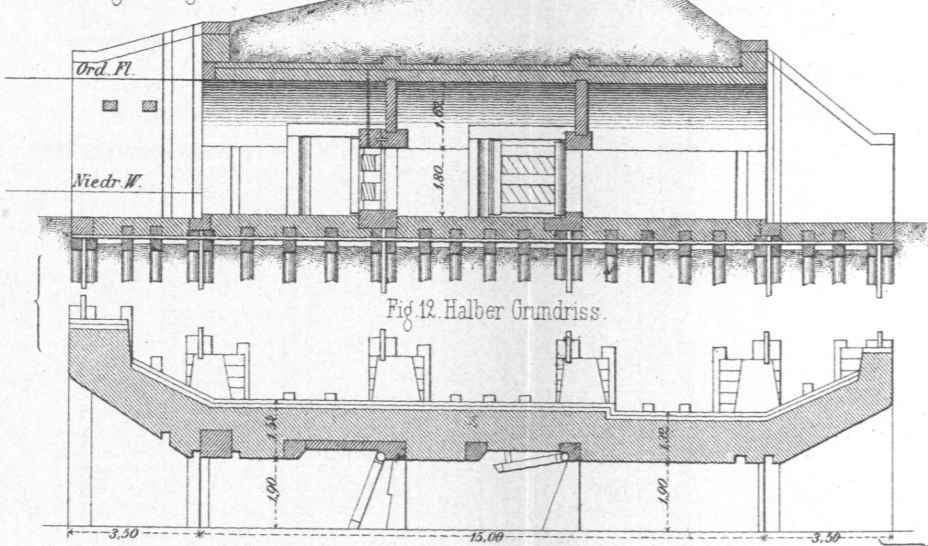
Maßstab zu Fig. 11 bis 14: 0,005.
