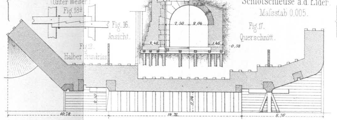
Fig. 19 bis 21. Deichschleuse am Dollart. (Statensiel.)
