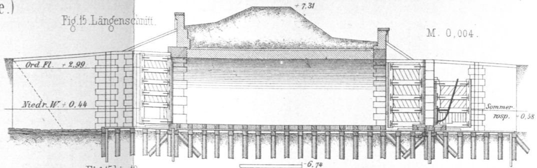
Fig. 15 bis 18. Aschwardener Siel. (Unter Weser.)
