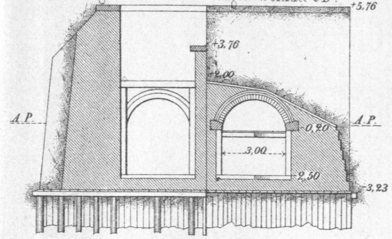
Fig. 3. Längenschnitt.
