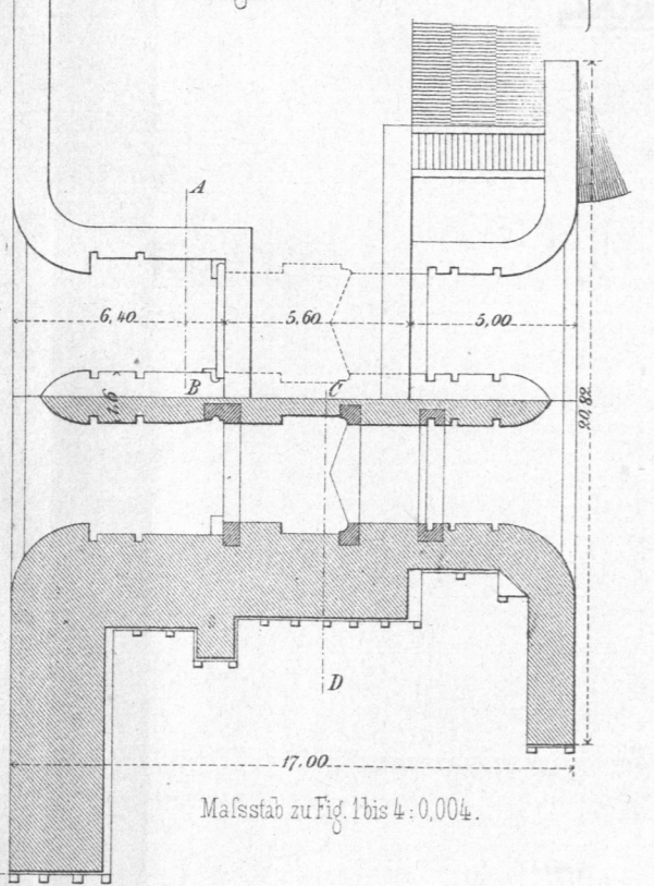
Fig. 4. Grundriss.
