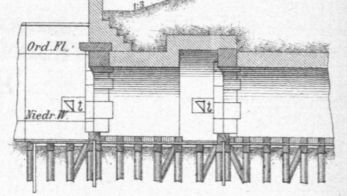
Fig. 11. Längenschnitt.
