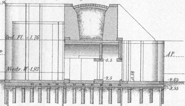
Fig. 3. Längenschnitt.
